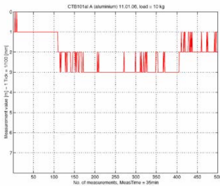
Figure 4c - trépied en alu Leica GST103
