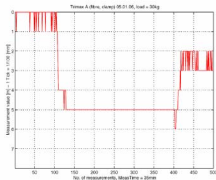
Figure 3c - trépied en fibre de verre Crain Trimax
