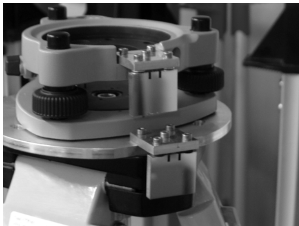
Figure 2 - miroirs d'autocollimation montés sur le trépied et l'embase pour la détection de déformations rotatoires.
