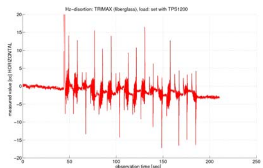
Figure 5c - trépied en fibre de verre Crain Trimax
